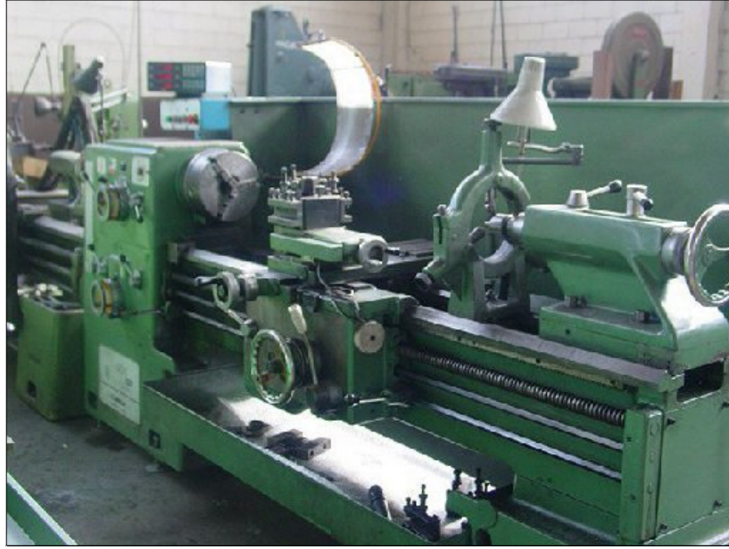
TORNIO PARALLELO
